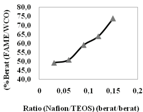
Gambar 3. Hubungan produk biodisel (% berat) dan konsentrasi Nafion dalam Nafion/TEOS.
