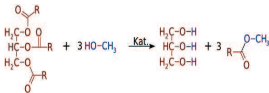
Gambar 2. Reaksi transesterifikasi minyak dengan alkohol menghasilkan metal ester dan gliserol.
