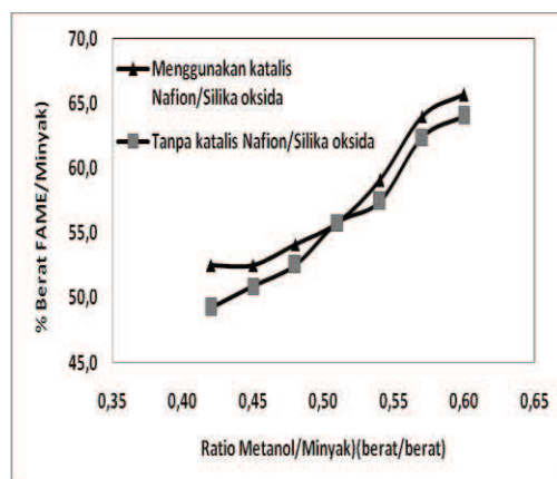
Gambar 4. Perbedaan % Berat biodisel dengan menggunakan katalis ganda dan katalis tunggal dengan perbandingan Metanol/minyak yang divariasasi.
