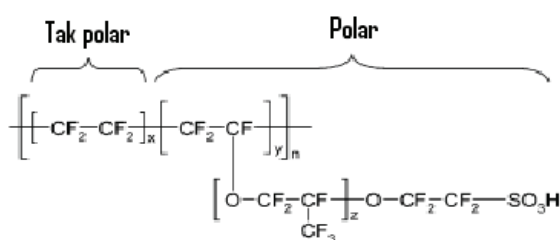
Gambar 1. Struktur Nafion.
