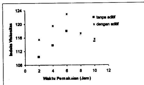
Gambar 6. Hubungan antara waktu pemakaian minyak pelumas dengan indeks viskositas
