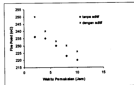
Gambar 8. Hubungan antara waktu pemakaian minyak pelumas dengan fire point .
