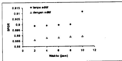
Gambar 5. Hubungan antara waktu pemakaian minyak pelumas dengan specipic gravity .
